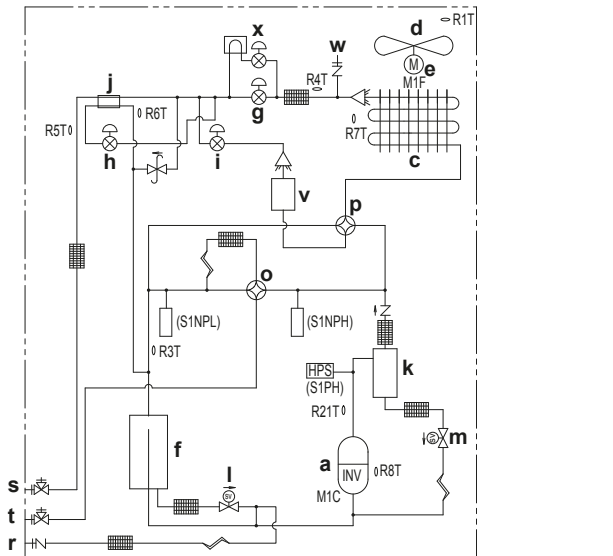
Схема трубопроводов: RYYQ8~12
